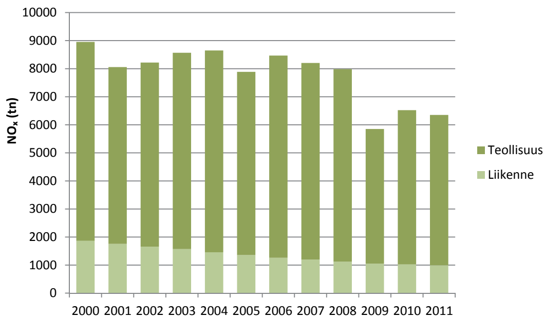
Kuva 5. Tutkimusalueen lupavelvollisten laitosten ja liikenteen typen oksidien päästöt (tn/v) vuosina 2000–2011 (Ympäristöhallinnon VAHTI-tietojärjestelmä 2012, LIISA 2011).
