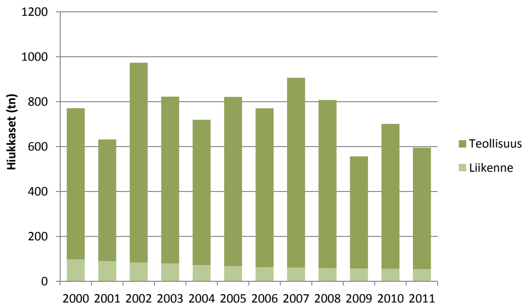
Kuva 6. Tutkimusalueen lupavelvollisten laitosten ja liikenteen hiukkaspäästöt (tn/v) vuosina 2000–2011 (Ympäristöhallinnon VAHTI-tietojärjestelmä 2012, LIISA 2011).
