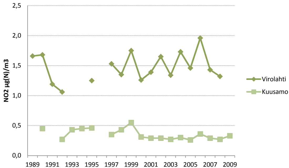
Kuva 15. Typpidioksidin pitoisuus typpinä ( \mu\text{g N/m}^3 ) ilmassa Virolahden ja Kuusamon tausta-aseilla vuosina 1989–2009, vuosikeskiarvot (Salmi 2009, Salmi 2011a).
