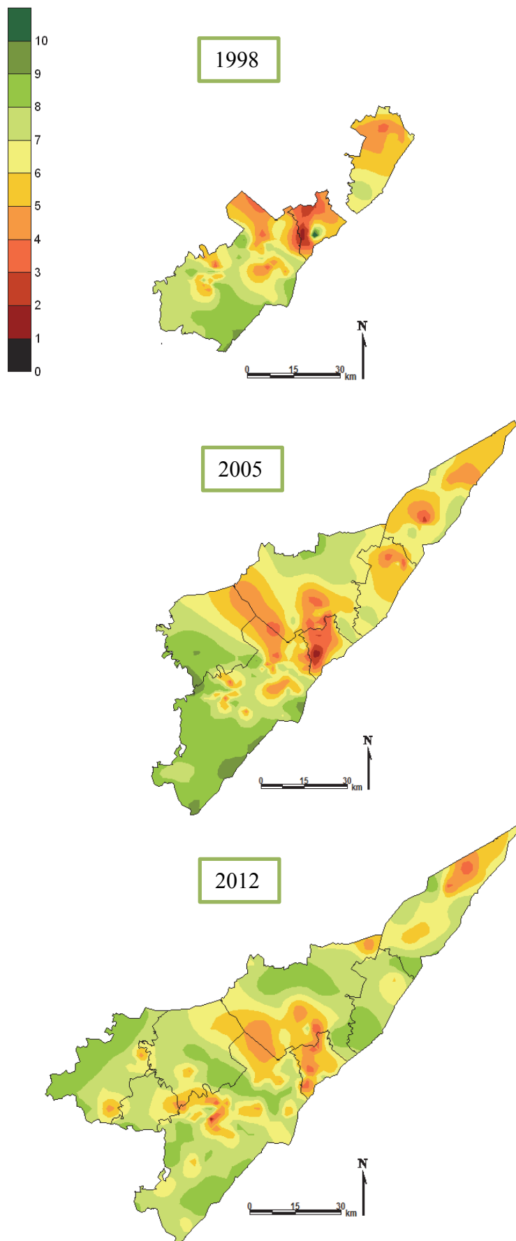
Kuva 53. Ilman epäpuhtausista kärsivien jäkälien lukumäärät havaintoaloilla vyöhykkeittäin 1998, 2005 ja 2012.
