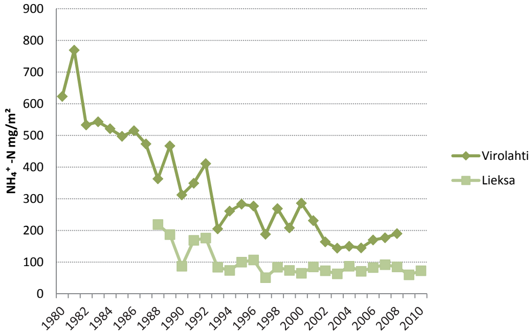
Kuva 18. Ammoniumityypen vuosilaskeumat ( \text{NH}_4^+ -N \text{mg}/\text{m}^2 ) Virolahden ja Lieksan Hietajärven mittausasemilla vuosina 1980-2010 (Salmi 2009, Salmi 2011b).
