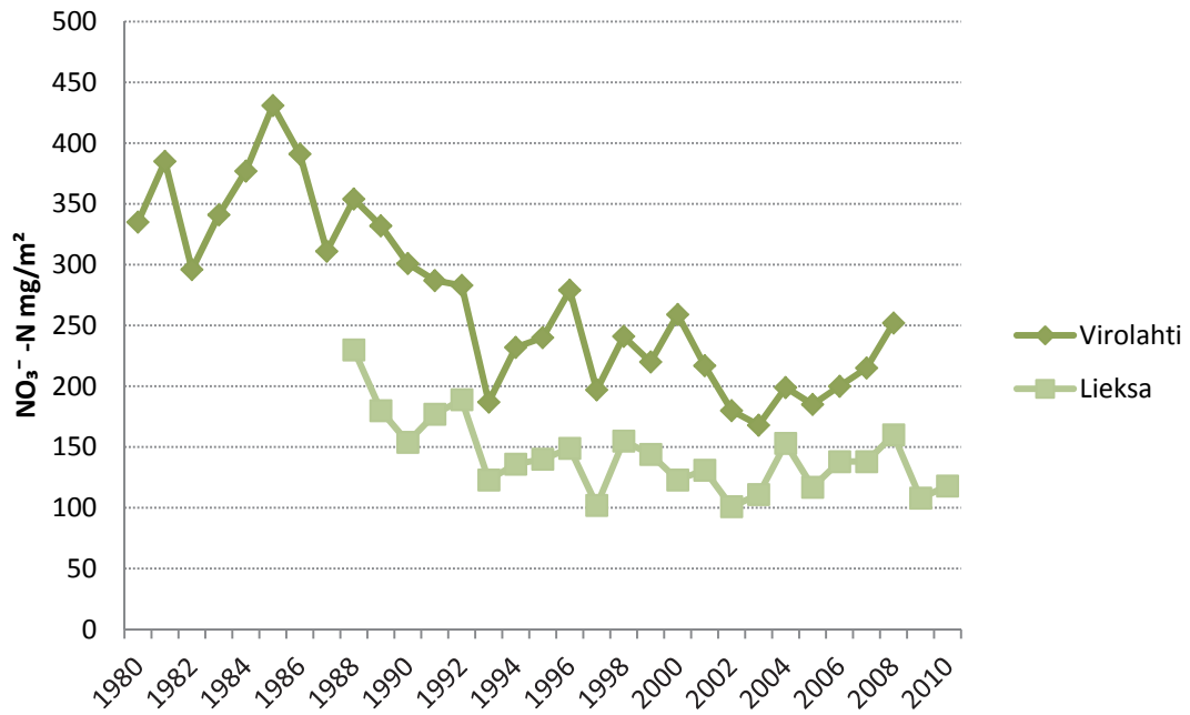
Kuva 17. Nitraattityypen vuosilaskeumat ( \text{NO}_3^- -N \text{mg}/\text{m}^2 ) Virolahden ja Lieksan Hietajärven mittausasemilla vuosina 1980-2010 (Salmi 2009, Salmi 2011b).
