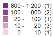
Rikkidioksidin päästöt (tn) kunnittain vuonna 2010
